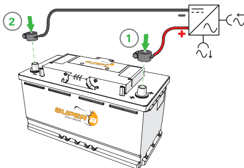
Abbildung 12. Anschluss von Stromkabeln mit Kraftfahrzeug-Anschlussklemmen und Kappen
