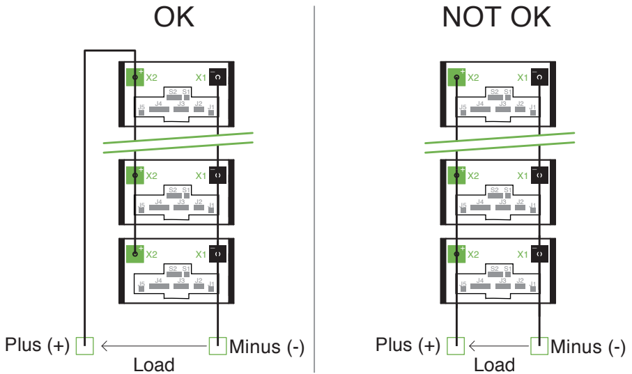
Abbildung 17. Parallelanschluss der Batterien
