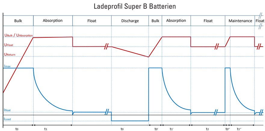
Abbildung 18. Ladekurve
