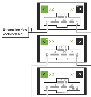
Abbildung 15. Beispiel für den Anschluss der Datenkabel von 3 Batterien mit einer externen Schnittstelle (3x CAT5e FTP-Netzwerk, 2x RJ45-Abschlussvorrichtungen)
