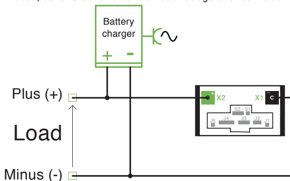
Abbildung 16. Anschluss eines Ladeegerätes an die Batterie
