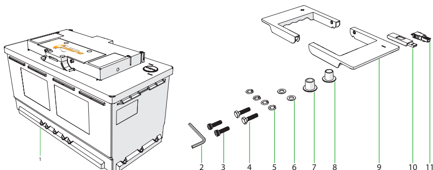
Abbildung 2. Komponenten
