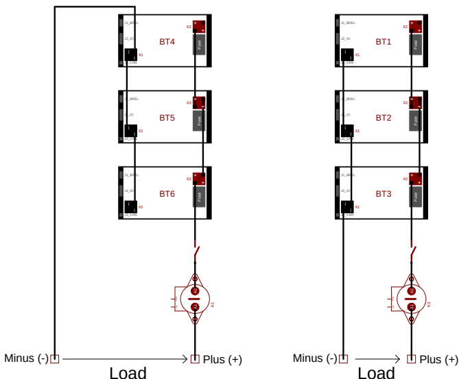
Abbildung 15. Drei mit einem externen Relais parallel angeschlossene Li-ion-Batterien
