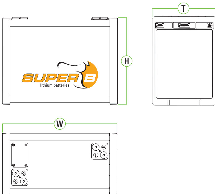
Abbildung 1. Abmessungen
