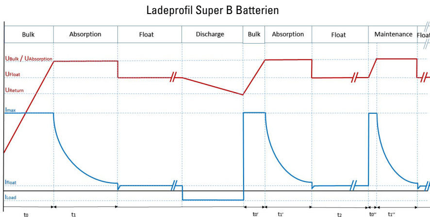
Abbildung 19. Ladekurve
